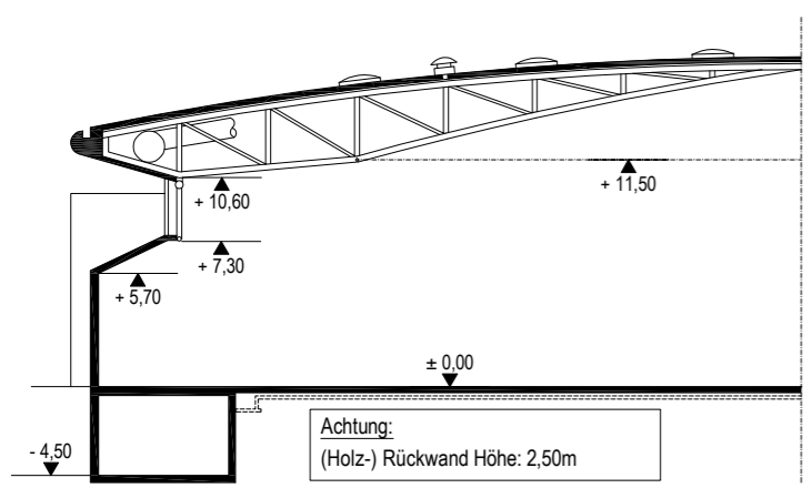
SCHNITT
